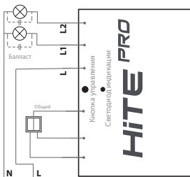
Схема подключения выключателя к блоку радиореле HITE PRO Relay-F2 с установкой блока в подрозетнике за выключателем
