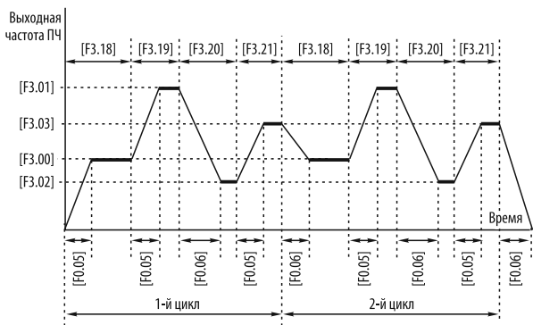
Рисунок 56 – циклический режим программы ПЛК.
