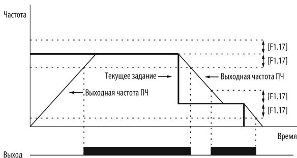
Рисунок 43 – включение дискретного выхода при достижении частоты текущего задания.
