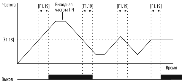
Рисунок 44 – включение дискретного выхода при достижении предустановленной частоты [F1.18].
