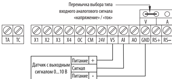
Рисунок 19 – схема подключения датчика с аналоговым выходным сигналом 0...10 В (питание от встроенного источника питания 10 В).
