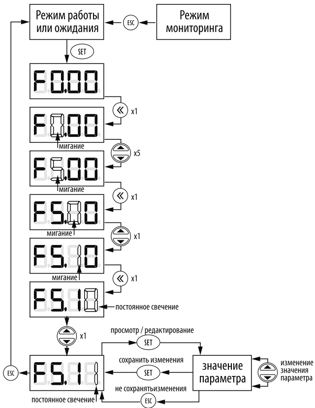
Рисунок 33 – быстрый переход к параметрам в режиме программирования
