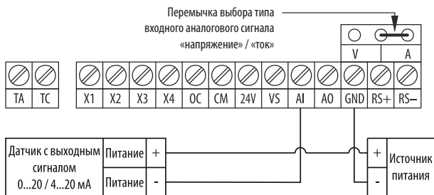
Рисунок 18 – схема подключения 2-х проводного датчика с аналоговым выходным сигналом 0...20 / 4...20 мА (питание от внешнего источника питания).
