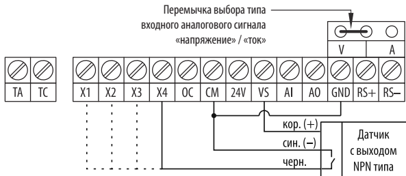
Рисунок 13 – Схема подключения датчиков с выходом NPN типа к дискретным входам (питание от встроенного источника питания 10 В).
