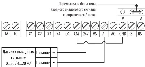
Рисунок 17 – схема подключения 2-х проводного датчика с аналоговым выходным сигналом 0...20 / 4...20 мА (питание от встроенного источника питания 24 В).
