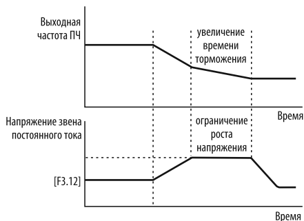
Рисунок 51 – ограничение роста напряжения в звене постоянного тока.
