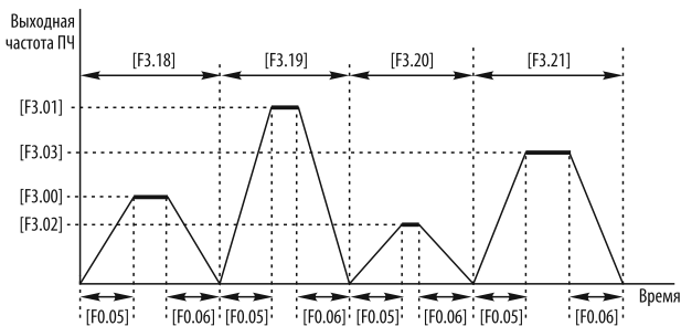
Рисунок 53 – режим программы ПЛК «Один цикл с остановом между скоростями».
