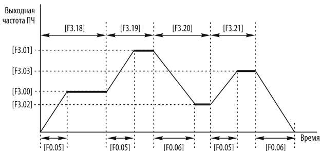
Рисунок 52 – режим программы ПЛК «Один цикл без остановки между скоростями».
