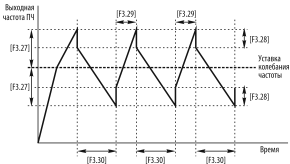
Рисунок 57 – работа ПЧ в режиме колебания частоты.
