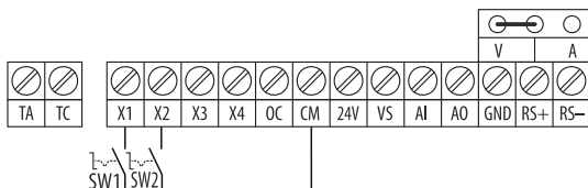
Рисунок 34 - подача команд «Пуск/Стоп» с дискретных входов (двухпроводная схема)
