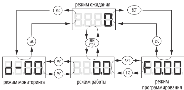
Рисунок 29 – переход между режимами работы ПЧ.
