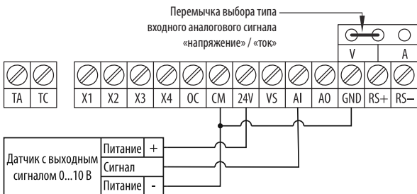
Рисунок 20 – схема подключения датчика с аналоговым выходным сигналом 0...10 В (питание от встроенного источника питания 24 В).
