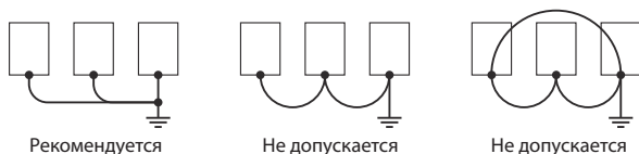
Рисунок 9 – рекомендуемая схема заземления нескольких ПЧ.
