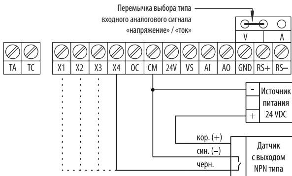
Рисунок 14 – Схема подключения датчиков с выходом NPN типа к дискретным входам (питание от внешнего источника питания).
