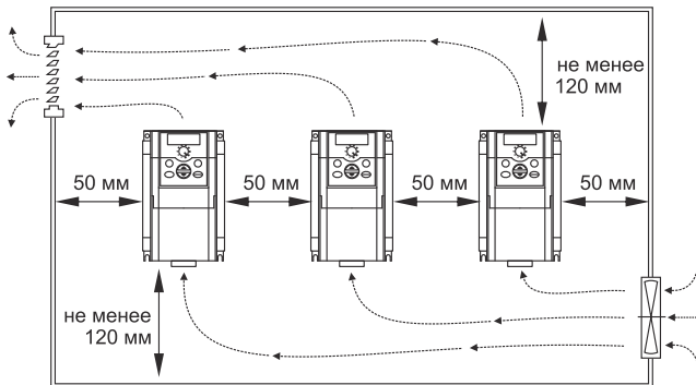
Рисунок 7 – Установка нескольких преобразователей частоты в одном шкафу.
