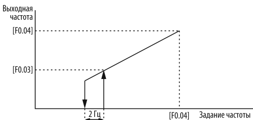
Рисунок 40 – переход ПЧ на нулевую частоту при текущем задании ниже нижнего предела
