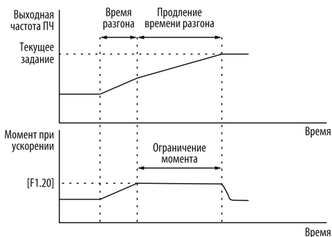
Рисунок 48 – ограничение момента при ускорении.
