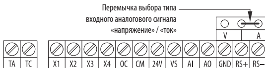
Рисунок 10 – Клеммы цепей управления.
