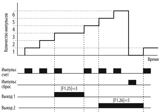
Рисунок 46 – работа встроенного счетчика импульсов.
