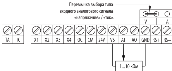
Рисунок 15 – схема подключения внешнего потенциометра.
