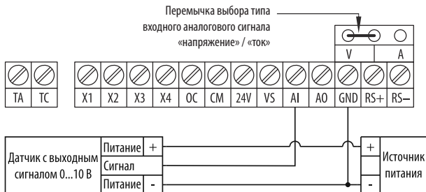
Рисунок 21 – схема подключения датчика с аналоговым выходным сигналом 0...10 В (питание от внешнего источника питания).
