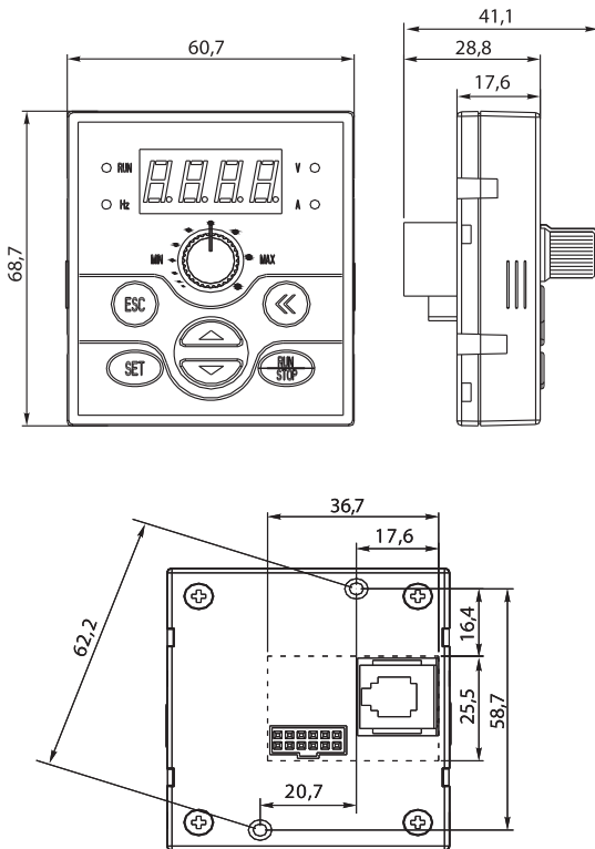
Рисунок 8 – габаритные и установочные размеры панели управления.
