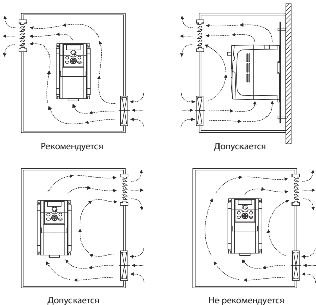
Рисунок 6 – Расположение элементов системы дополнительной вентиляции.
