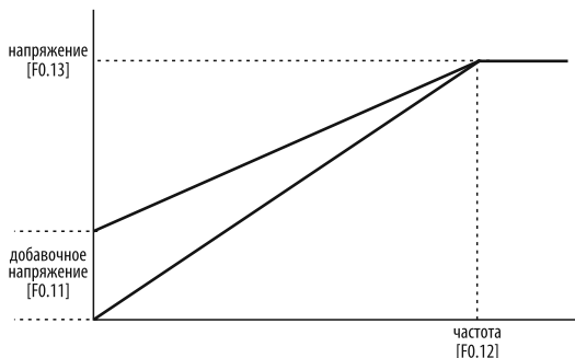
Рисунок 38– добавочное напряжения электродвигателя в функции усиления момента.
