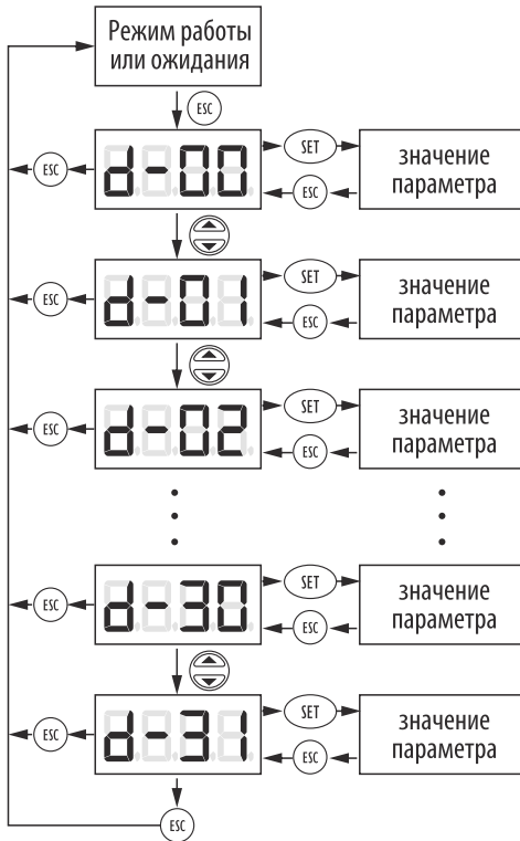
Рисунок 31 – меню ПЧ в режиме мониторинга
