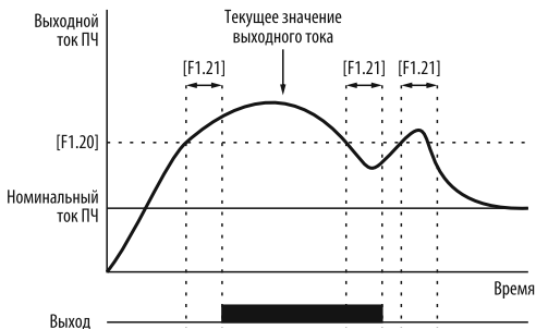
Рисунок 45 – включение дискретного выхода при обнаружении перегрузки ПЧ по току.
