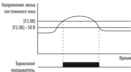
Рисунок 49 – динамическое торможение ПЧ.
