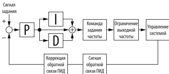
Рисунок 58 – работа ПИД-регулятора.
