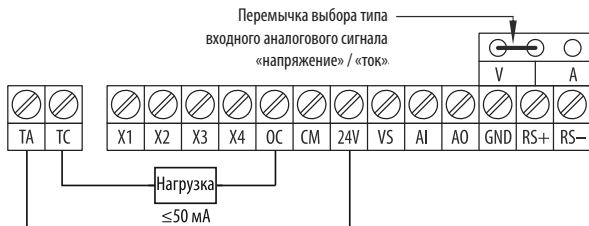
Рисунок 22 – схема подключения нагрузки к релейному выходу (питание от встроенного источника питания 24 В).
