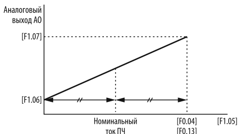
Рисунок 42 – соответствие минимального и максимального значений выходного сигнала АО выходному параметру ПЧ, назначенному в параметре [F1.05] .
