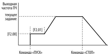
Рисунок 47 – работа ПЧ на начальной частоте.
