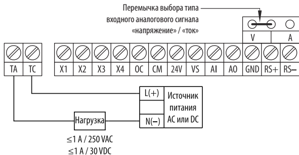
Рисунок 23 – схема подключения нагрузки к релейному выходу (питание от внешнего источника питания постоянного или переменного тока).
