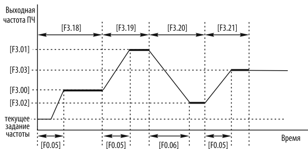
Рисунок 54 – режим программы ПЛК «Один цикл и работа на последней (четвертой) скорости».
