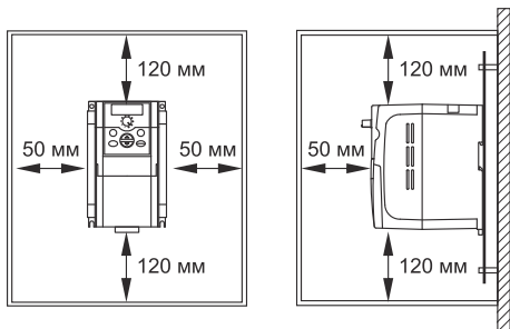
Рисунок 4 - Минимально допустимые расстояния от ПЧ до окружающих предметов.
