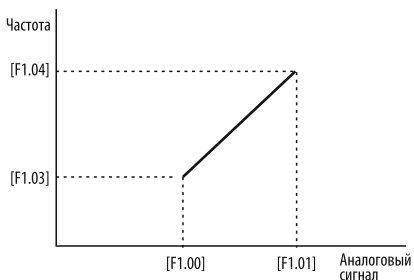
Рисунок 41 – зависимость выходной частоты от значения аналогового сигнала на входе AI.
