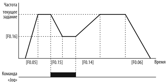
Рисунок 39 – работа ПЧ в режиме Jog.
