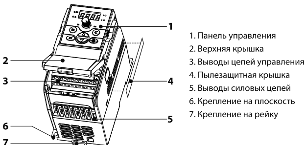
Рисунок 1 – корпус преобразователя частоты первого габарита
