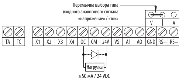
Рисунок 24 – схема подключения нагрузки к транзисторному выходу (питание от встроенного источника питания 24 В).
