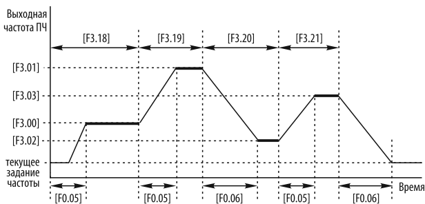
Рисунок 55 – режим программы ПЛК «Один цикл и работа на скорости текущего задания».
