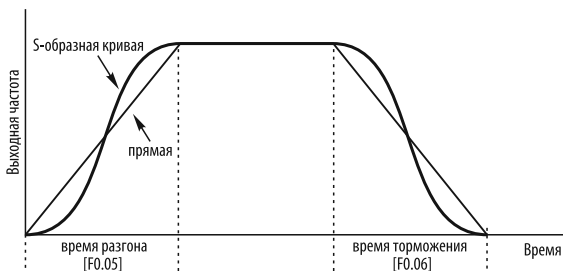
Рисунок 37 – характер разгона и торможения электродвигателя.
