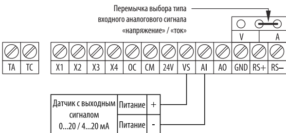
Рисунок 16 – схема подключения датчика с активным выходным сигналом 0...20 / 4...20 мА (питание от встроенного источника питания 10 В).
