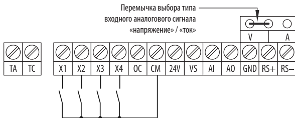
Рисунок 11 – Схема подключения сигнала типа «сухой контакт» к дискретным входам.
