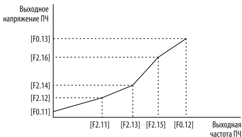
Рисунок 50 – пользовательская настройка U / f кривой.
