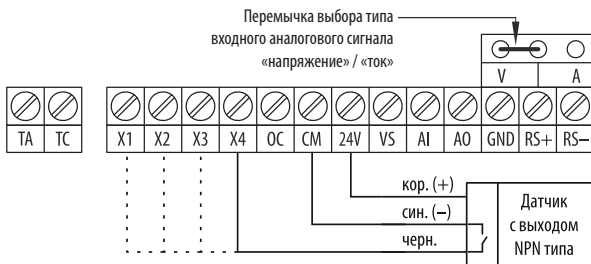
Рисунок 12 – Схема подключения датчиков с выходом NPN типа к дискретным входам (питание от встроенного источника питания 24 В).
