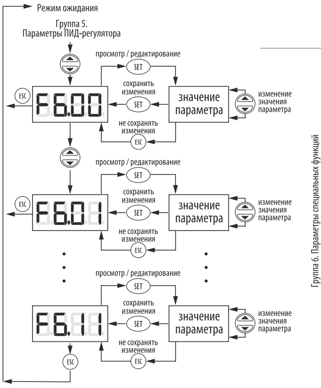
Рисунок 32 – меню ПЧ в режиме программирования (продолжение на следующей странице)
