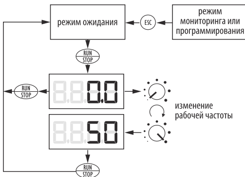
Рисунок 30 – меню ПЧ в режиме работы
