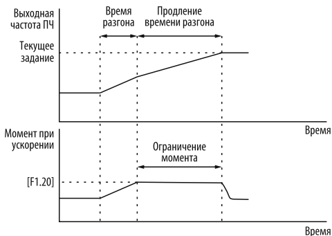
Рисунок 48 – ограничение момента при ускорении.
